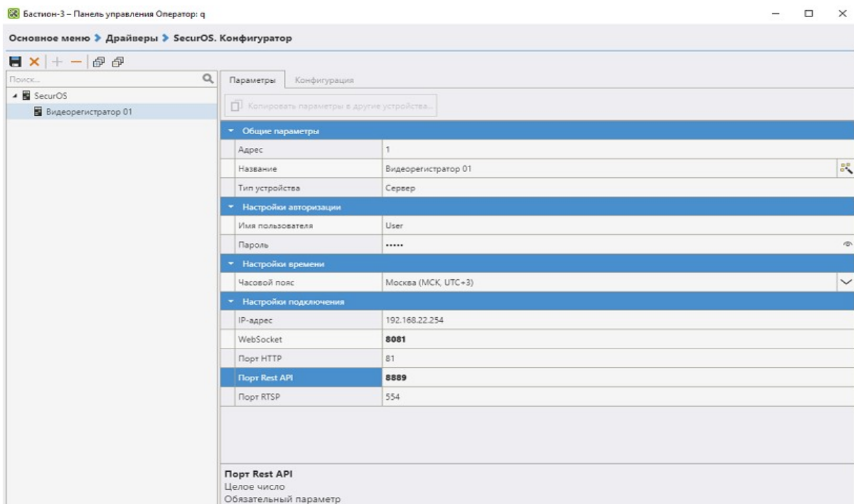
Рис. 9. Конфигуратор драйвера
